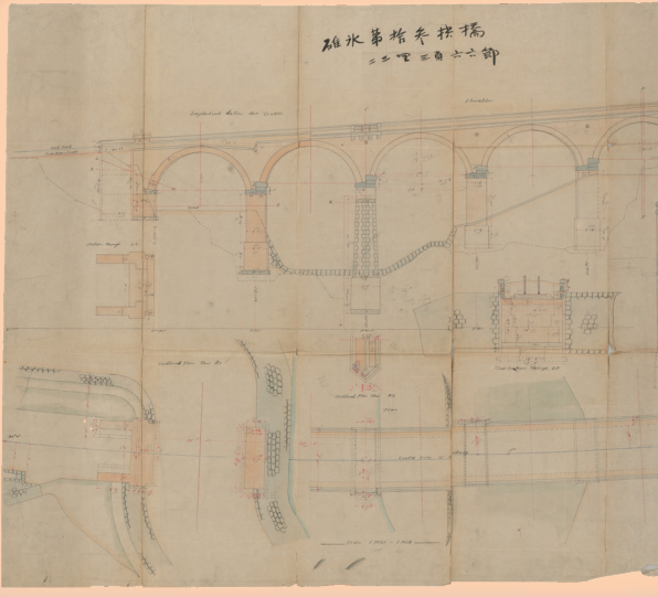
信越線（碓氷線）橋梁図面「碓氷第拾参拱橋」 安中市蔵
