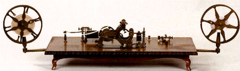
エンボッシング・モルルス電信機(ペリー-将来/米国製)(郵政博物館蔵)【国指定重要文化財】
